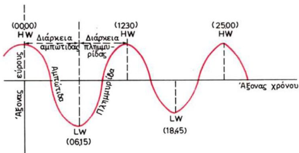
Σχ. 11.1δ. Παλιρροϊκό κύμα και στοιχεία του.
